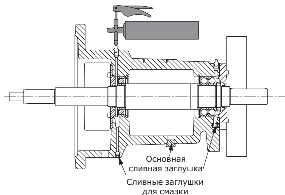
Рис. 28 Замена смазки
