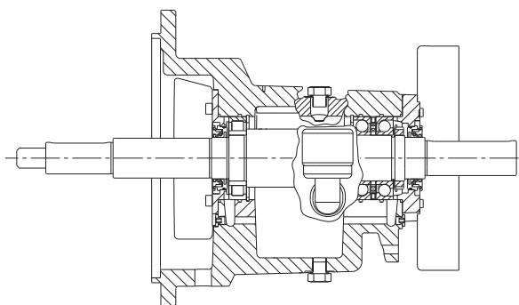
Рис. 29 Корпус с роликовыми и двойными радиально-упорными подшипниками с масляной смазкой
