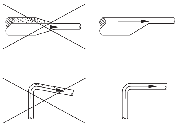
Рис. 10 Трубопроводы
