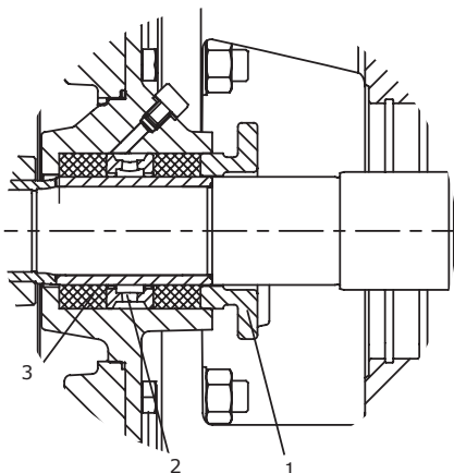
Рис. 24 Сальниковая букса в разрезе
