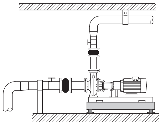
Рис. 11 Монтаж трубопровода
