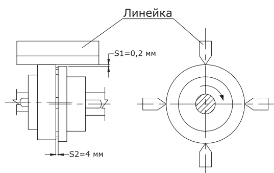
Рис. 9 Регулировка соосности
