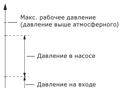
Рис. 31 Давление в насосе
