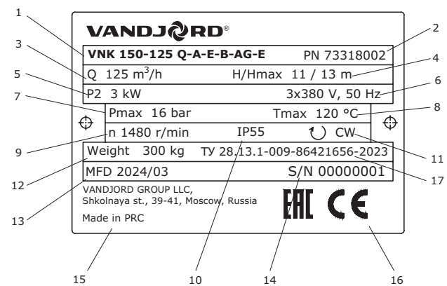
Рис. 2 Примеры фирменных табличек насосов
