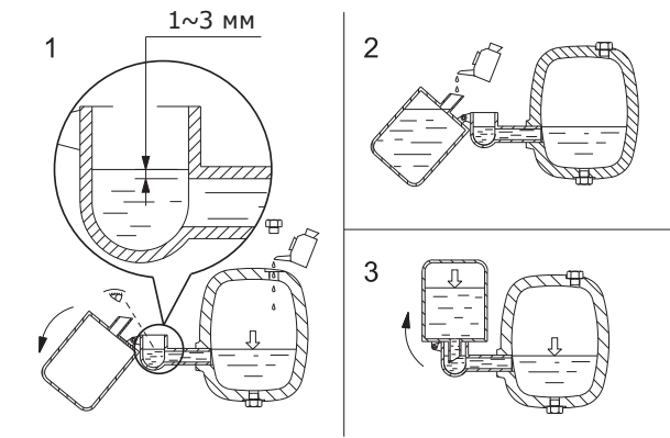
Рис. 17 Заливка масла
